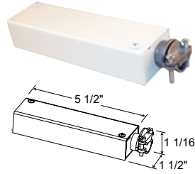
TL602E
