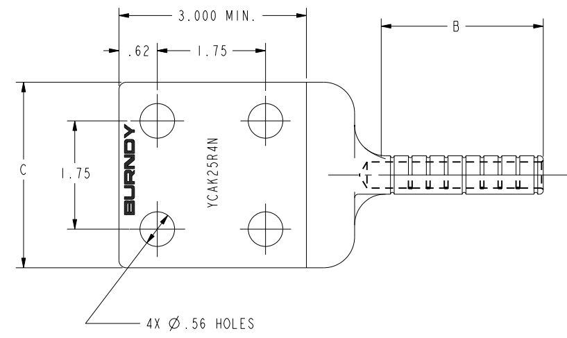
YCAK-R-4N FIG. 2
