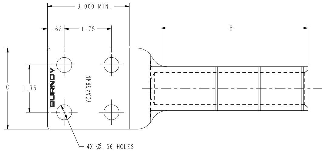
YCA-R-4N FIG. 3
